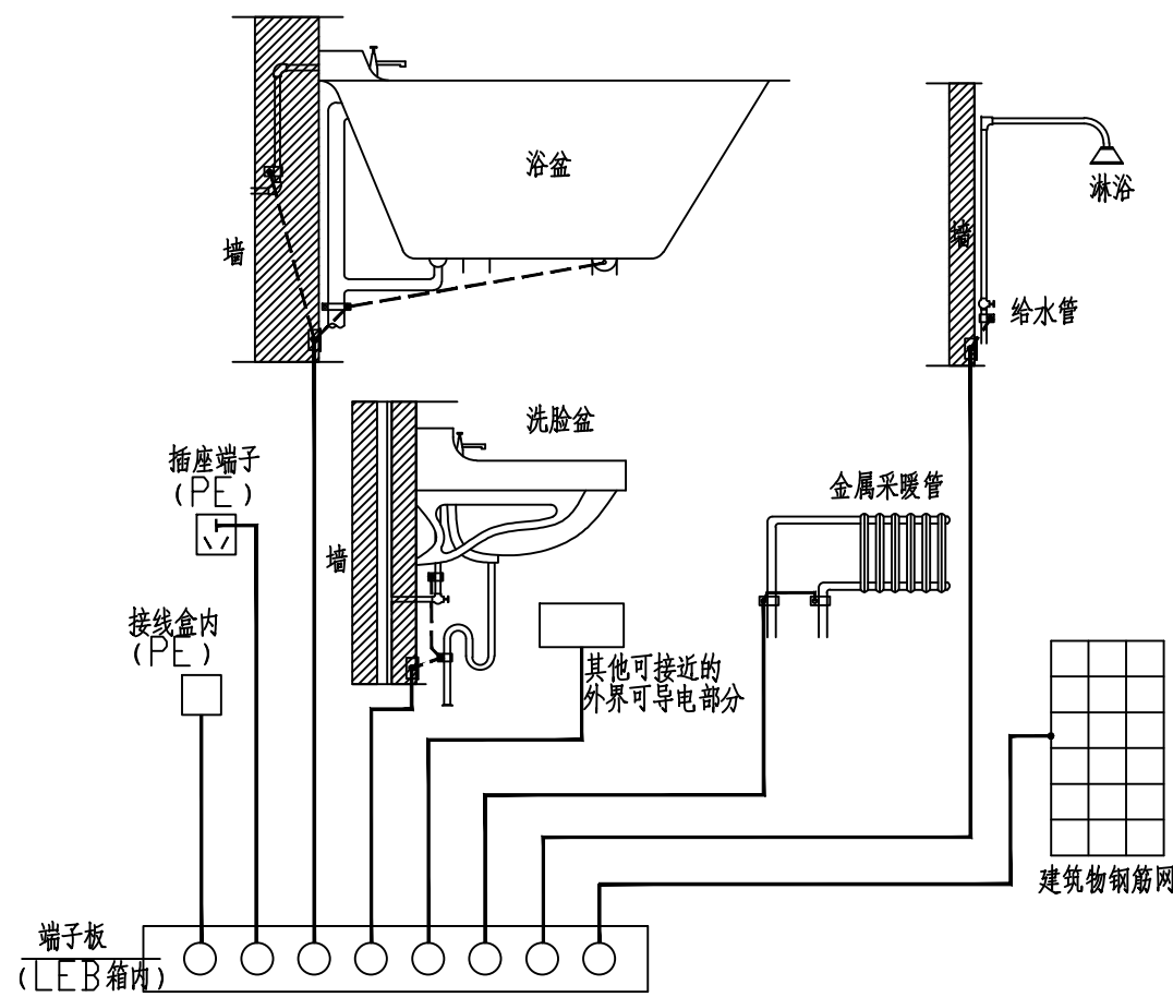
卫生间局部等电位连接做法
