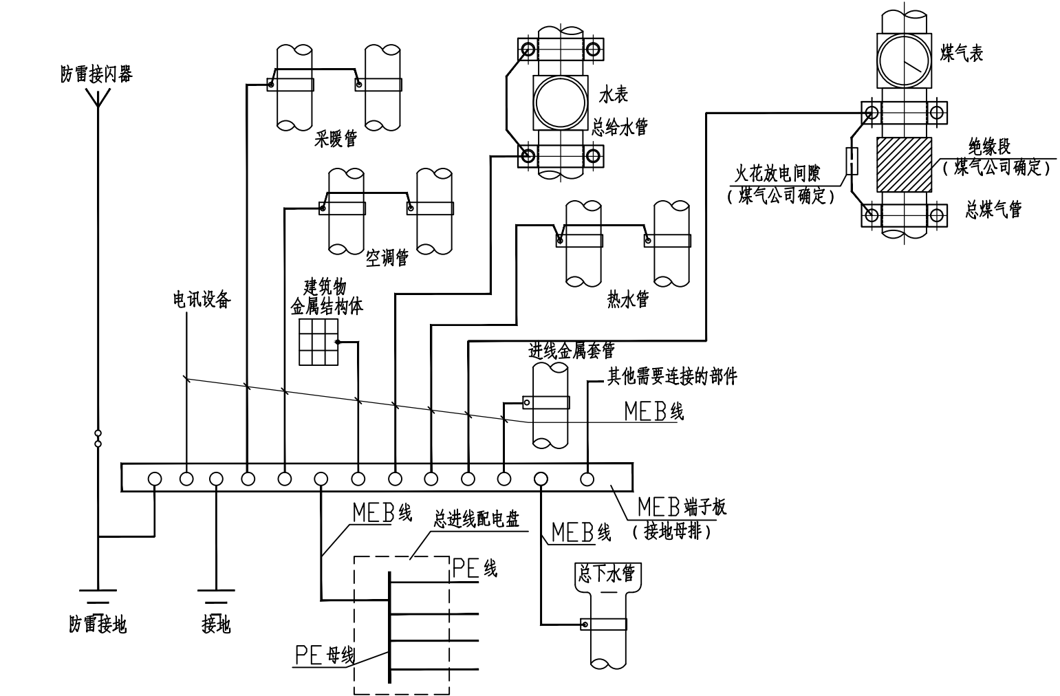
总等电位联结示意图
