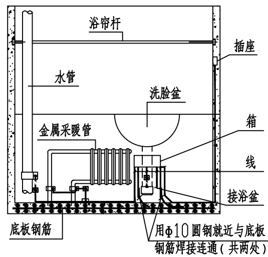
卫生间局部等电位剖面
